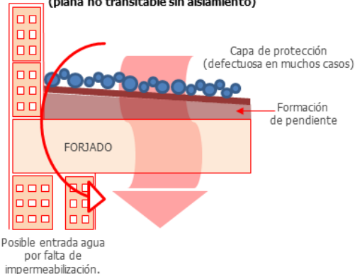
Ejemplo de defectos en cerramiento horizontal tipo (plana no transitable sin aislamiento)
